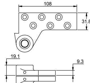
L180 top pivot
